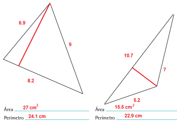
Figura 2. Area del Triangulo
